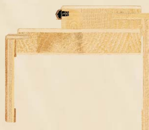
Telaio Olympia sezione traversa sup.
